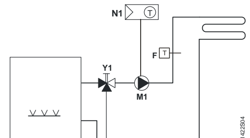
Regulace prostorové teploty přímým řízením oběhového čerpadla teplovodního podlahového vytápění.
