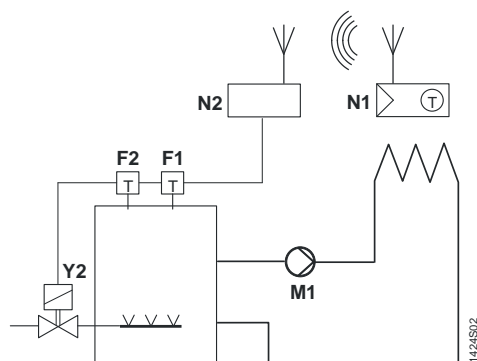
Bezdrátový regulátor a spínací jednotka regulují prostorovou teplotu přímým řízením závěsného plynového kotle.
