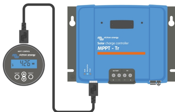
Připojení displeje k solární nabíječce pomocí kabelu VE.Direct
