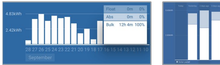
Vlevo: Příklad systému, který tráví veškerý čas v hromadné fázi. Vpravo: Rozdělení fázi nabíjení - systém tráví čas v objemové fázi a ve fázi absorpce.
