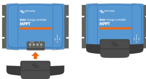
Příklad solární nabíječky s MPPT WireBox
