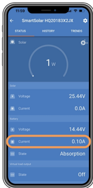
Aplikace VictronConnect ukazuje téměř nulový nabíjecí proud.
